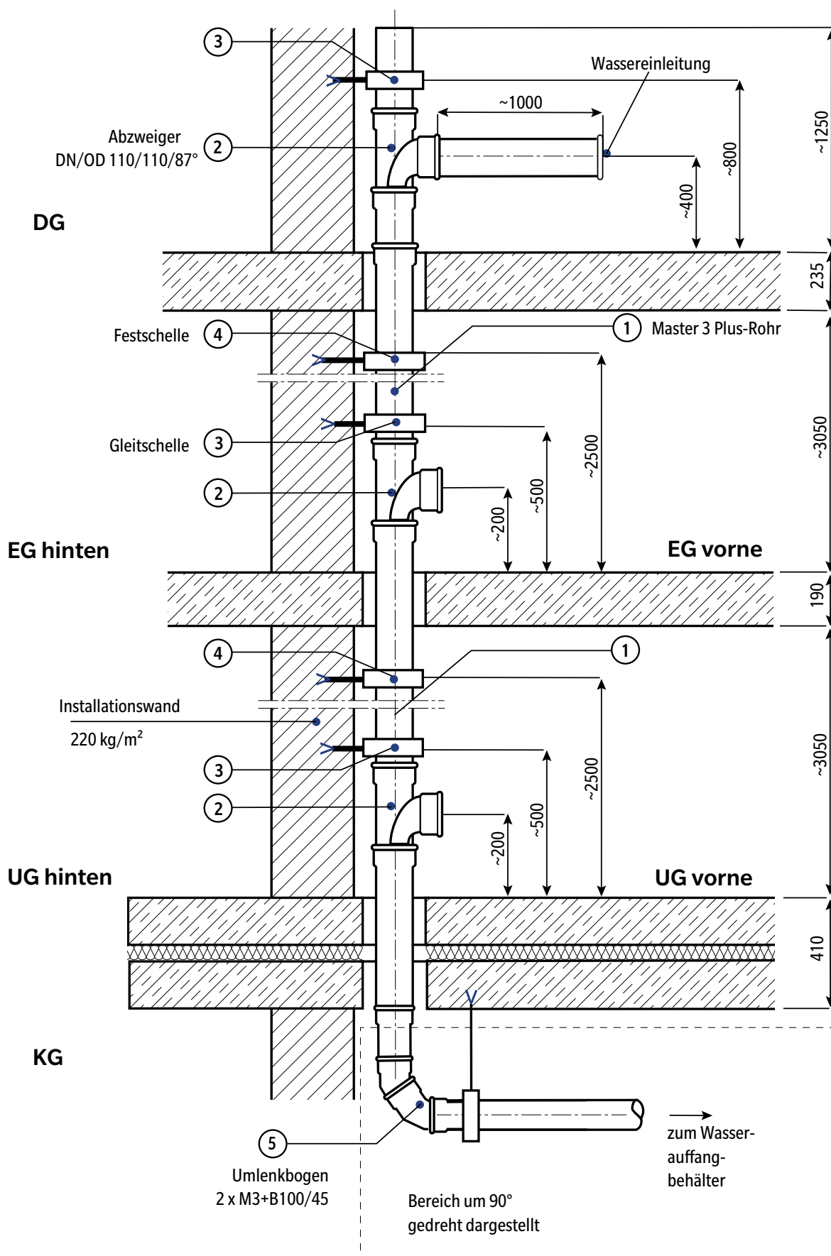
Abbildung1: Installationsplan der Schallmessungen für das Master3Plus-System am Fraunhofer-Institut in Stuttgart (nicht maßstabsgetreu, Abmessung in mm).
