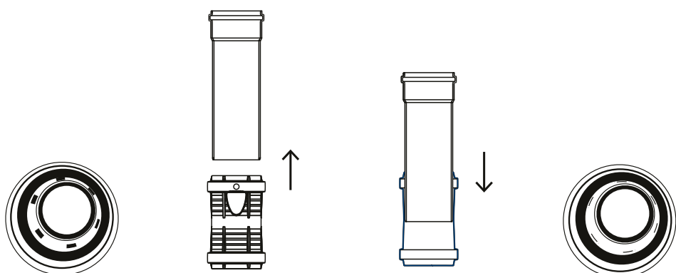
Überschubmuffe ohne Anschlagkanten
